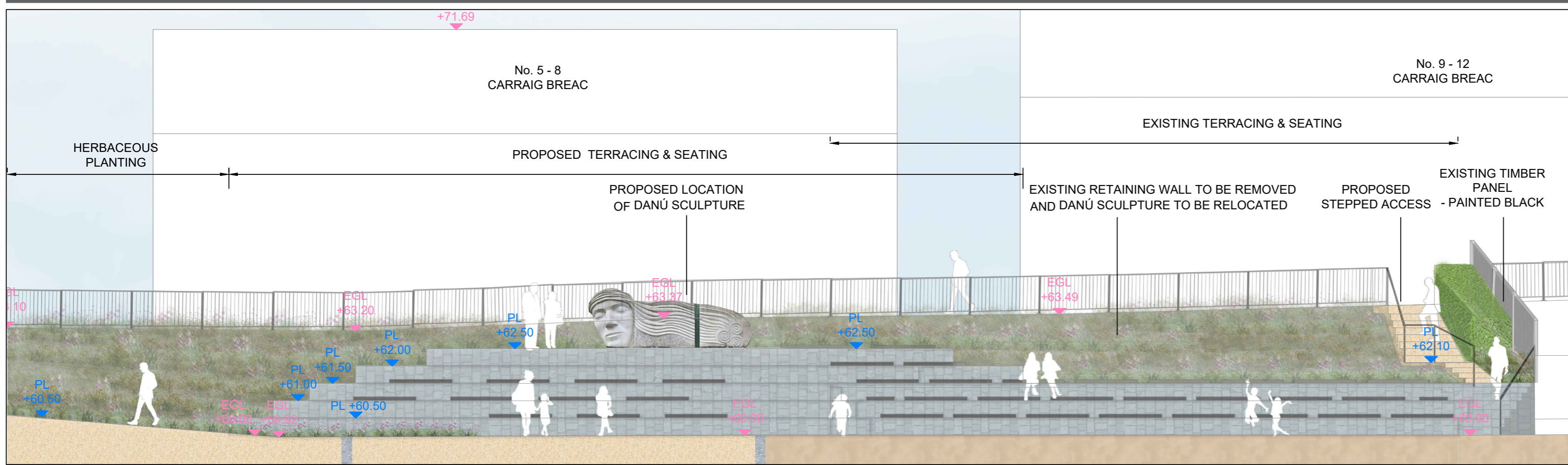
SECTION B-B - SCALE: 1:100 @A1
